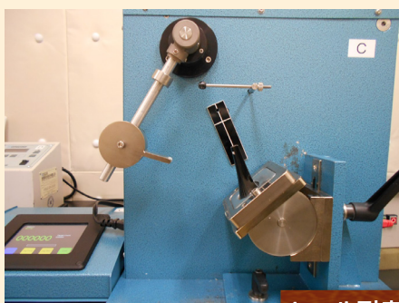
ヒール耐疲労性試験
