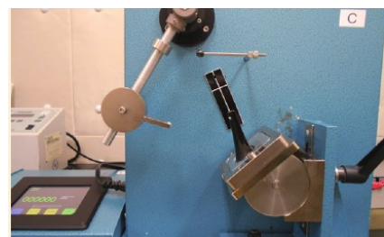
ヒール耐疲労性試験
